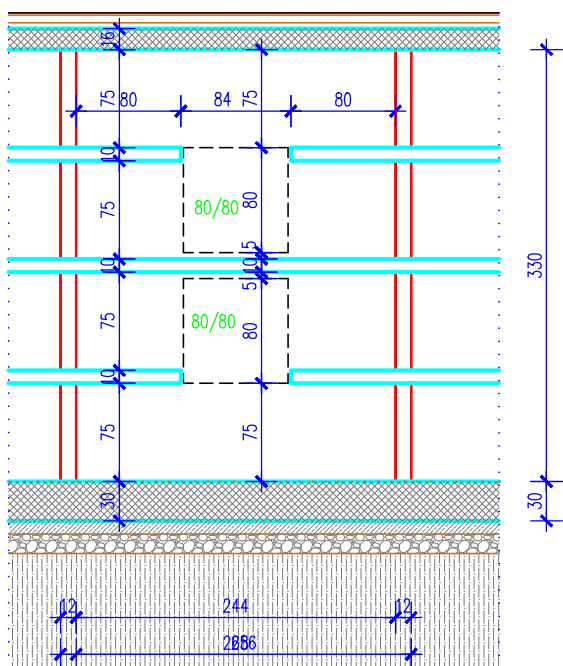
PRESJEK A-A
