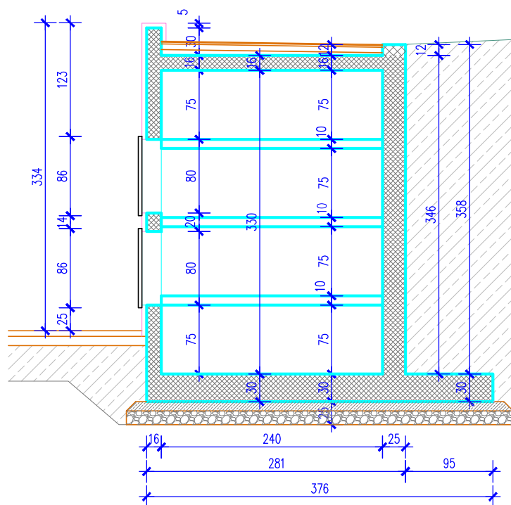
PRESJEK B-B
